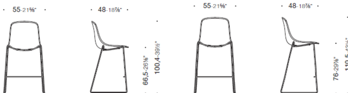
Shell, sgabello HS 66,5 con base a slitta lineare e schienale alto
