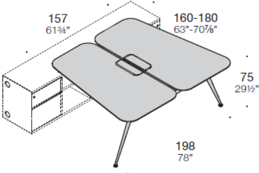
Piano trapezio per bench con top access pivot e vaschette
