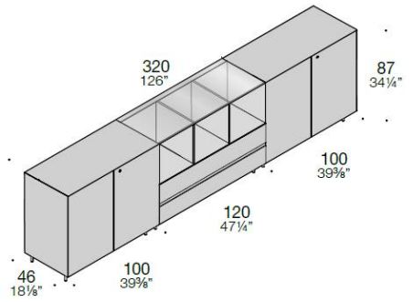
Contenitore L320 (1 modulo L120 + 2 moduli L100)
