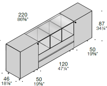
Contenitore L220 (2 moduli L50 + 1 modulo L120)
